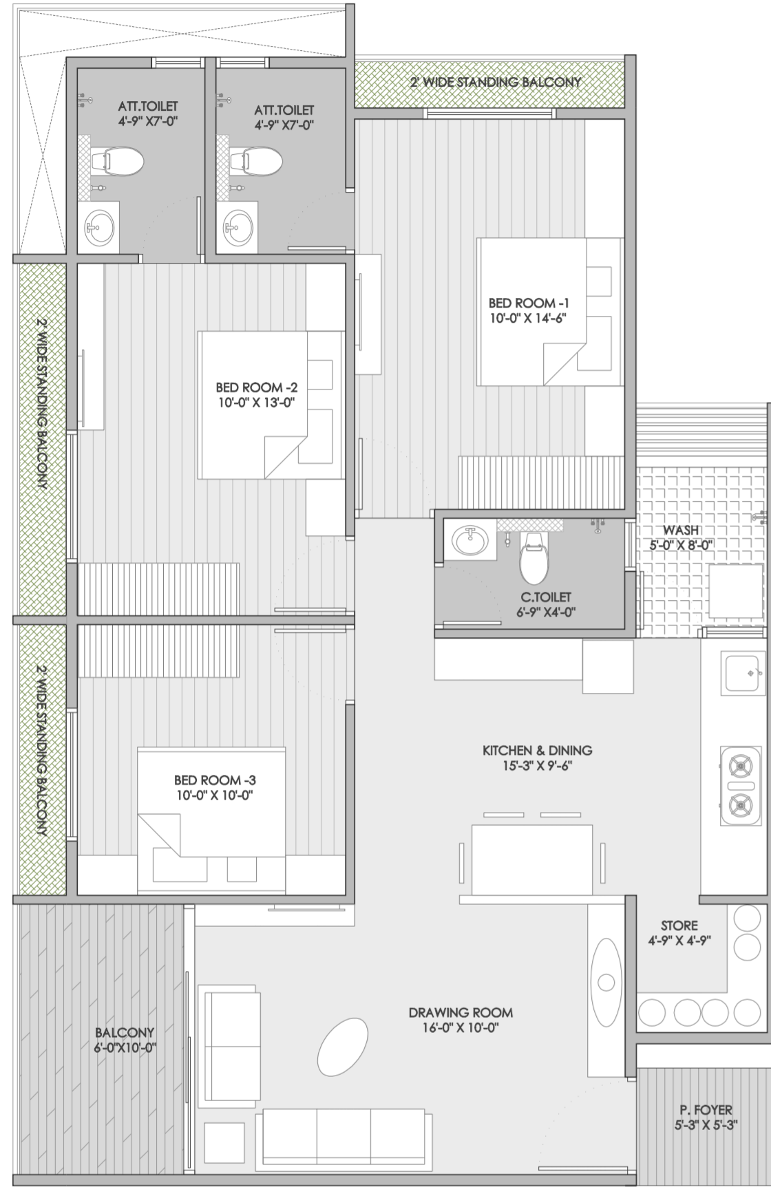
3BHK TYPE-1
